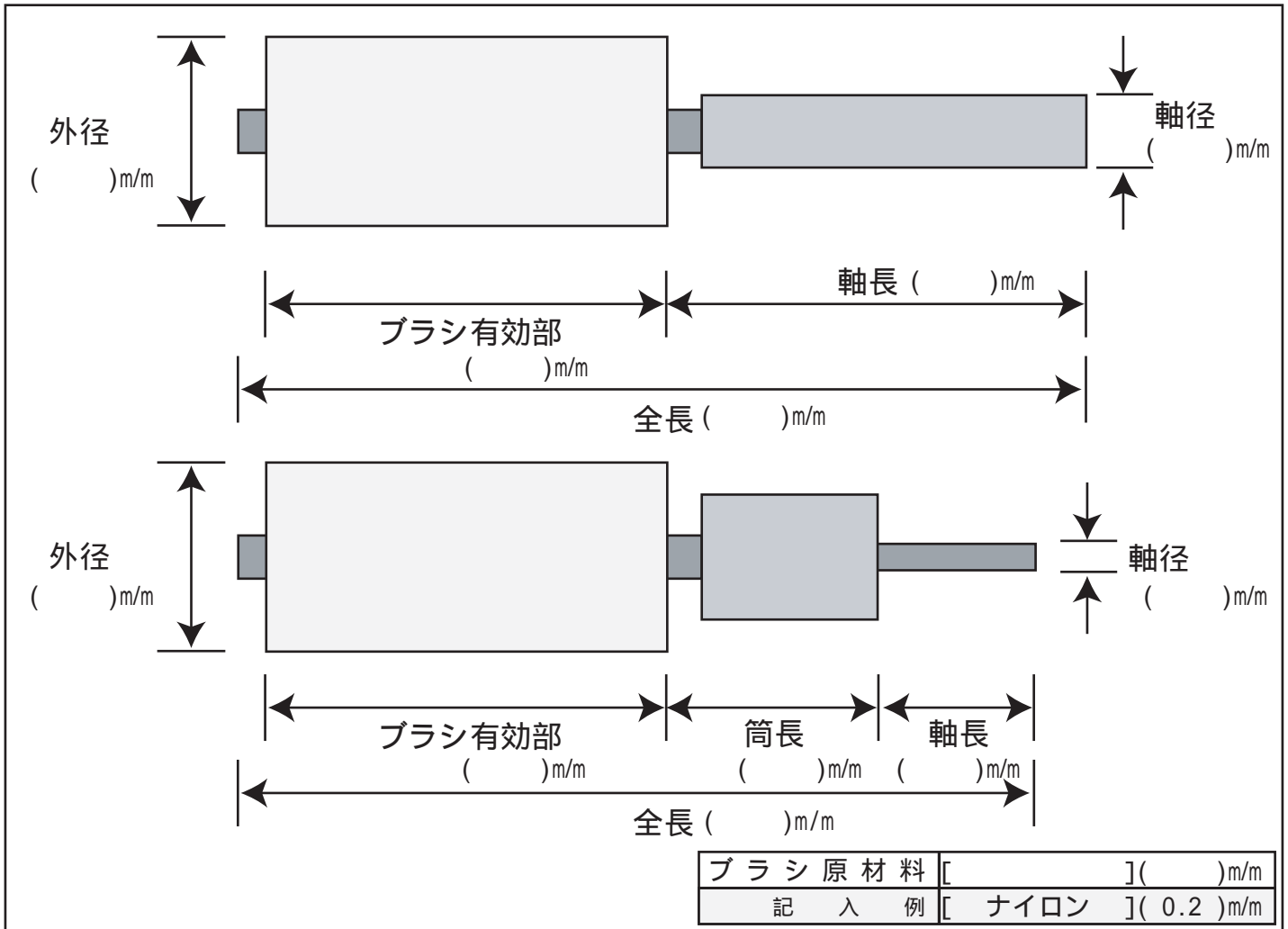
【シャンク付ねじりブラシ略図】
